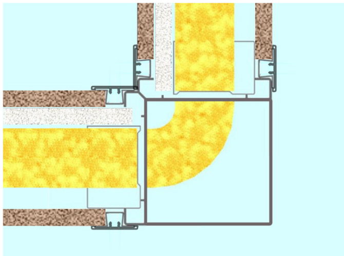
90° hoek
