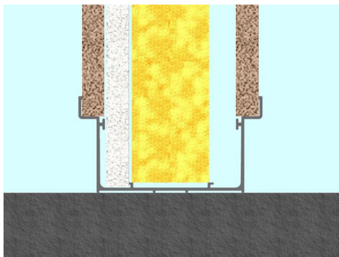
Aansluiting vloer
