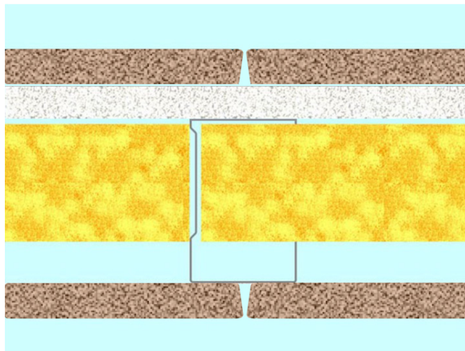
Koppeling gipsplaten
