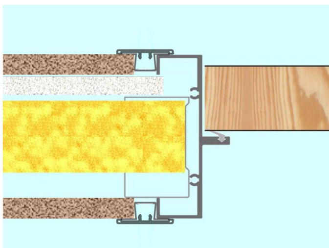
Aansluiting deurkozijn
