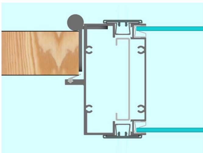
Aansluiting deurkozijn
