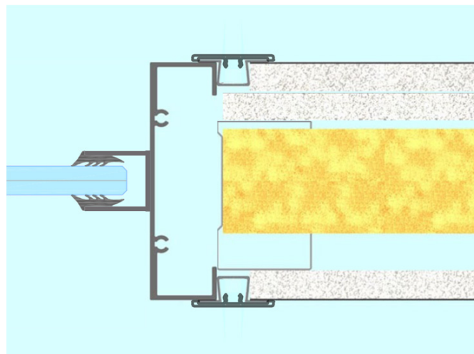
Aansluiting op enkel glas wand
