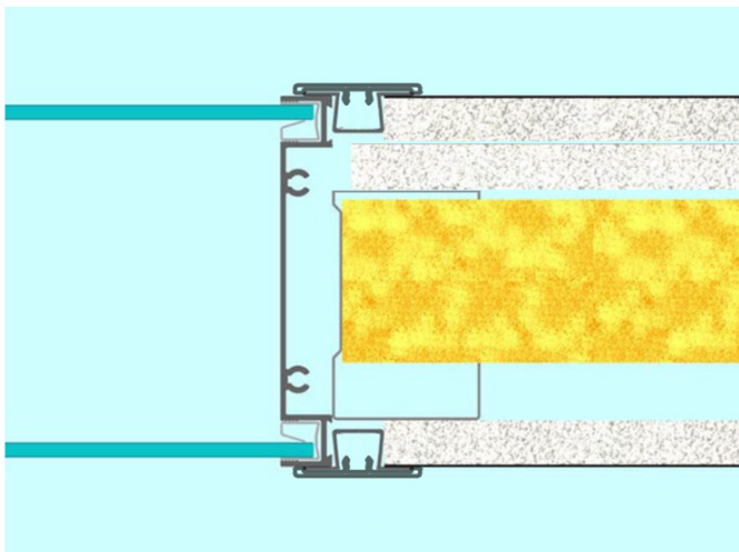
Aansluiting op dubbel glas wand
