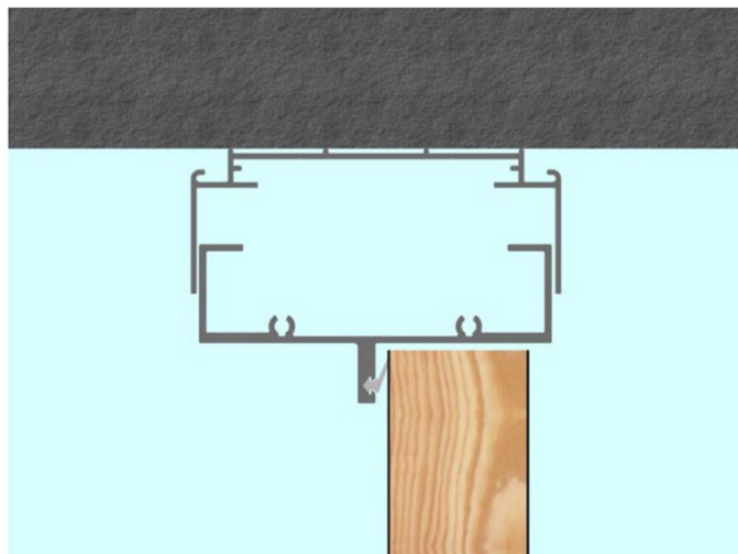
Aansluiting deurkozijn - plafond
